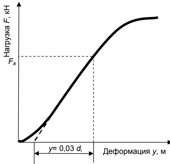
Рисунок В.1 – Кривая «нагрузка-деформация»
