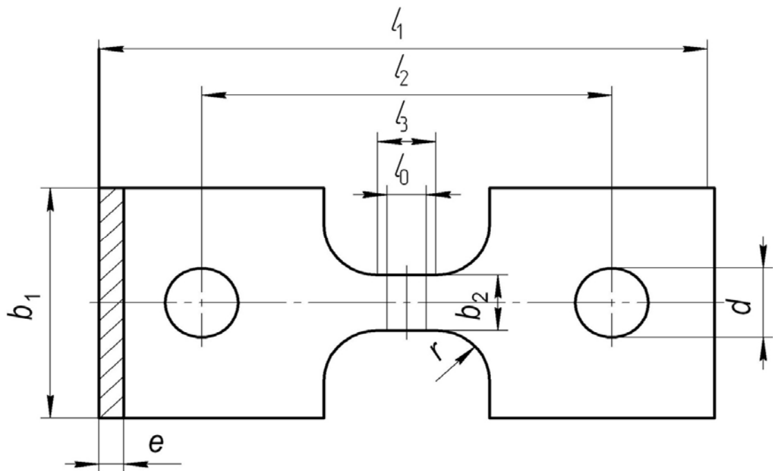
Рисунок 1 – Образец типа 3
