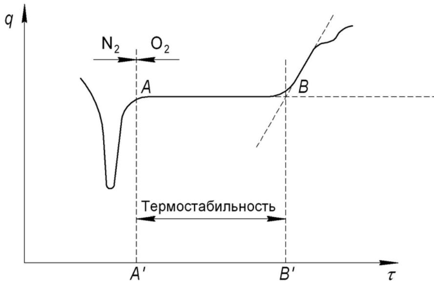
Рисунок Ж.1 – Типичная кривая ДСК при определении термоокислительной стабильности полиэтилена
