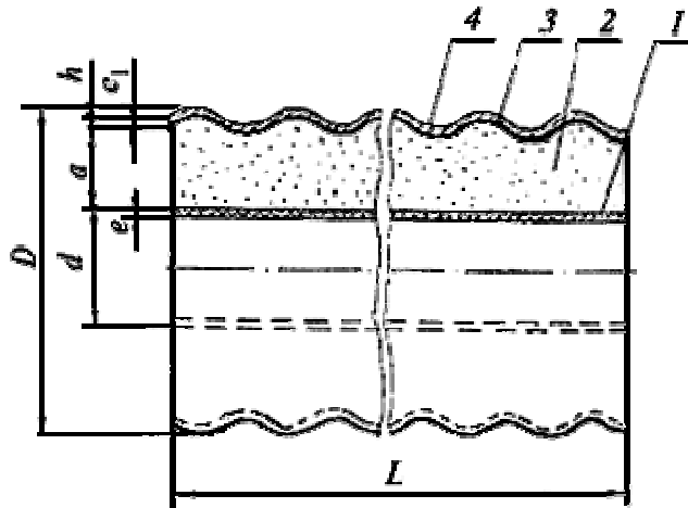
Рисунок 1 - Схема конструкции изолированных труб ПЭ-С
